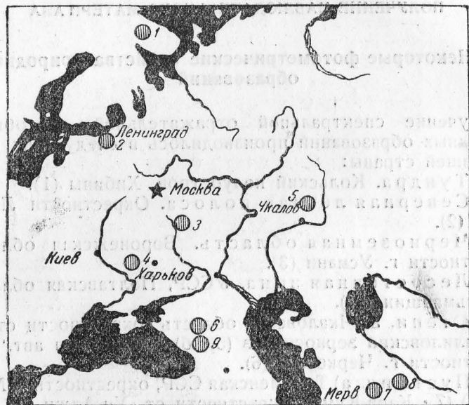
Фиг. 7. Схематическая карта районов полевых работ
