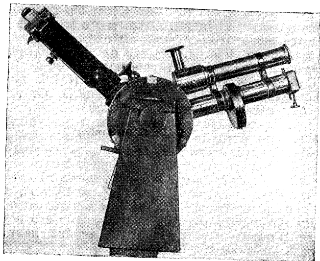
Фиг. 1. Полевой спектрограф НИЛ
